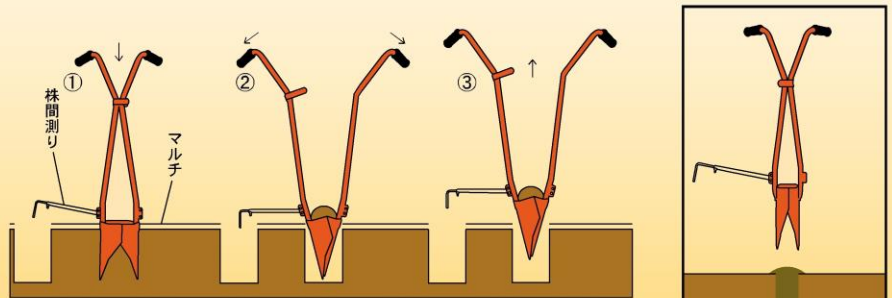
① ハンドルを閉じてクラウンを開き、株間測りで1つ前の穴との間隔を測りながら土中にさし込みます。 ② 土中でハンドルを開くとクラウンの中に土が入ります。 ③ ハンドルを開いてクラウンを開いたまま引き上げると穴があきます。 種芋の植え付けにも最適！
