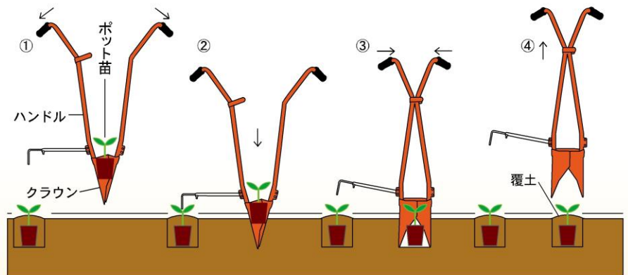
① ハンドルを開き、クラウン内にポット苗を入れます。 ② ハンドルを開いてクラウンを閉じたまま土中にさし込みます。 ③ 土中でハンドルを閉じてクラウンを開き、ポット苗を植え付けます。 ④ ハンドルを閉じてクラウンを開いたまま引き上げて土を覆います。
